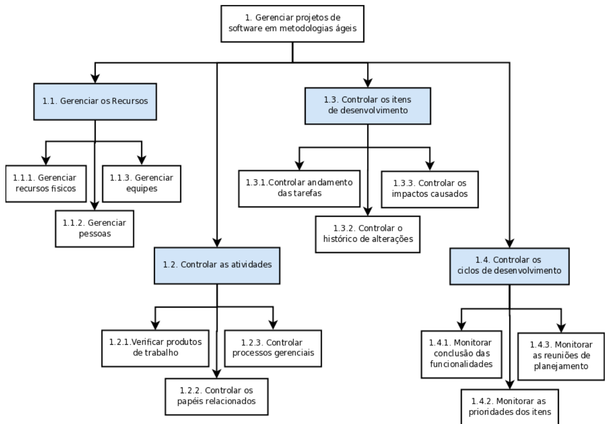
Figura 20: Objetivos do ambiente
