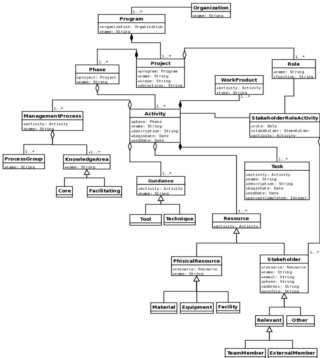
Figura 17: Metamodelo de gestão do PMBOK (Desenvolvido pelo autor)
