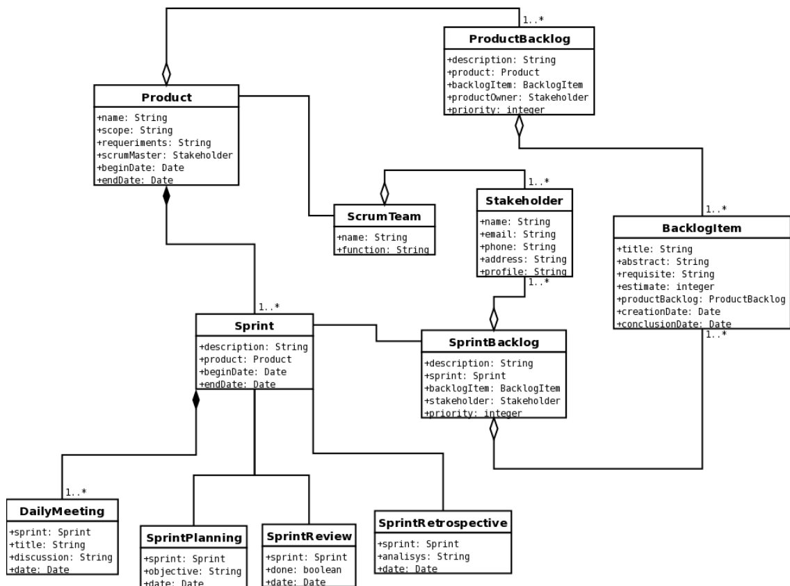
Figura 15: Metamodelo da metodologia Scrum (Desenvolvido pelo autor)
