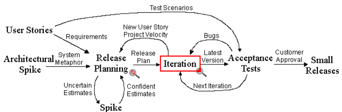
Figura 1: Processo da metodologia XP (XP, 2010)
