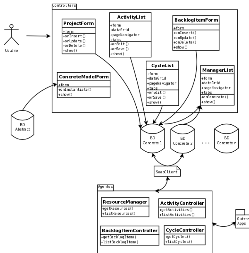
Figura 24: Arquitetura da aplicação
