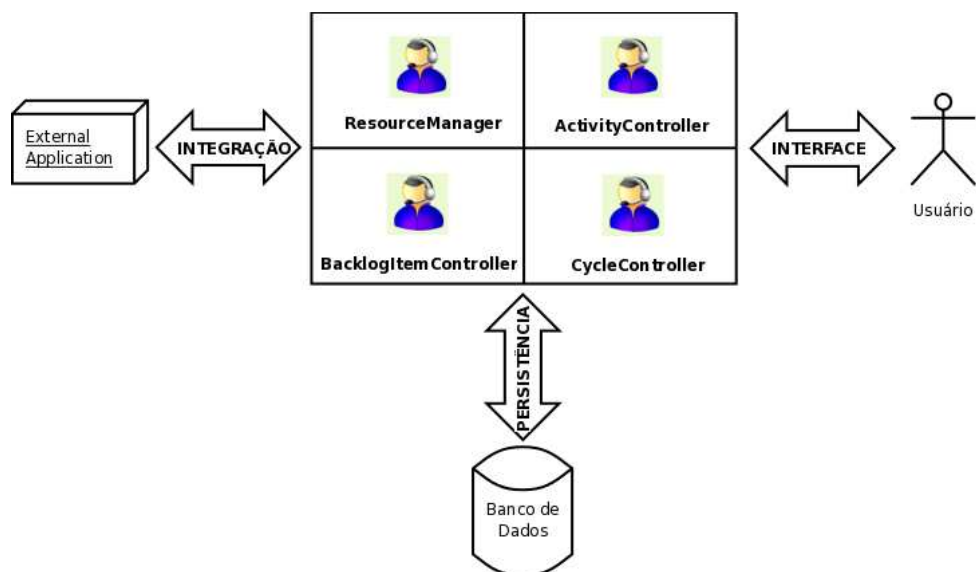
Figura 22: Arquitetura do ambiente
