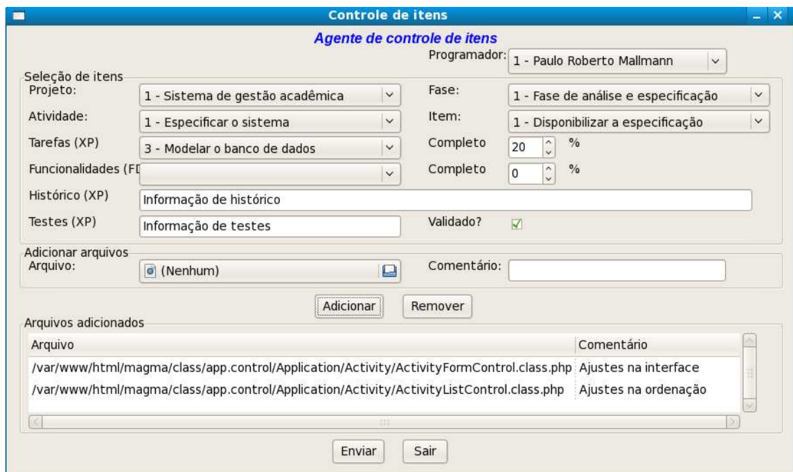
Figura 38: Interface do agente de itens
