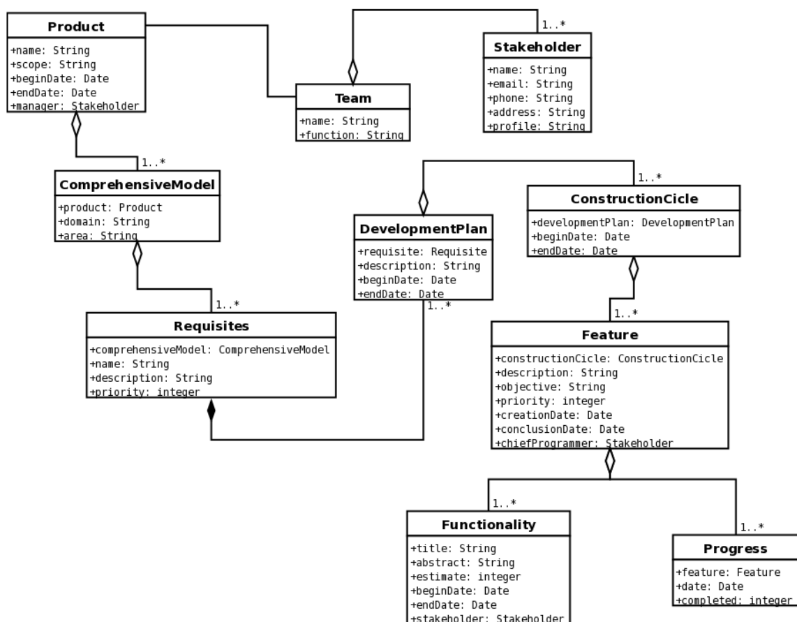
Figura 16: Metamodelo da metodologia FDD (Desenvolvido pelo autor)
