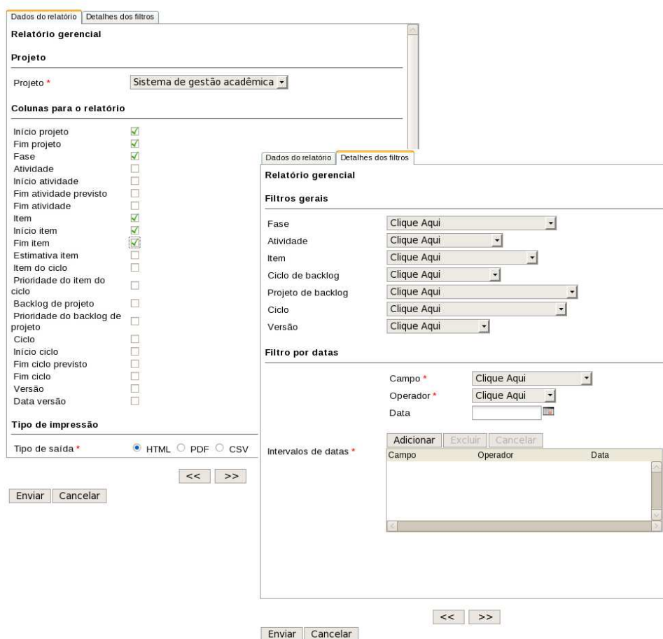
Figura 40: Interface de parametrização de um relatório gerencial
