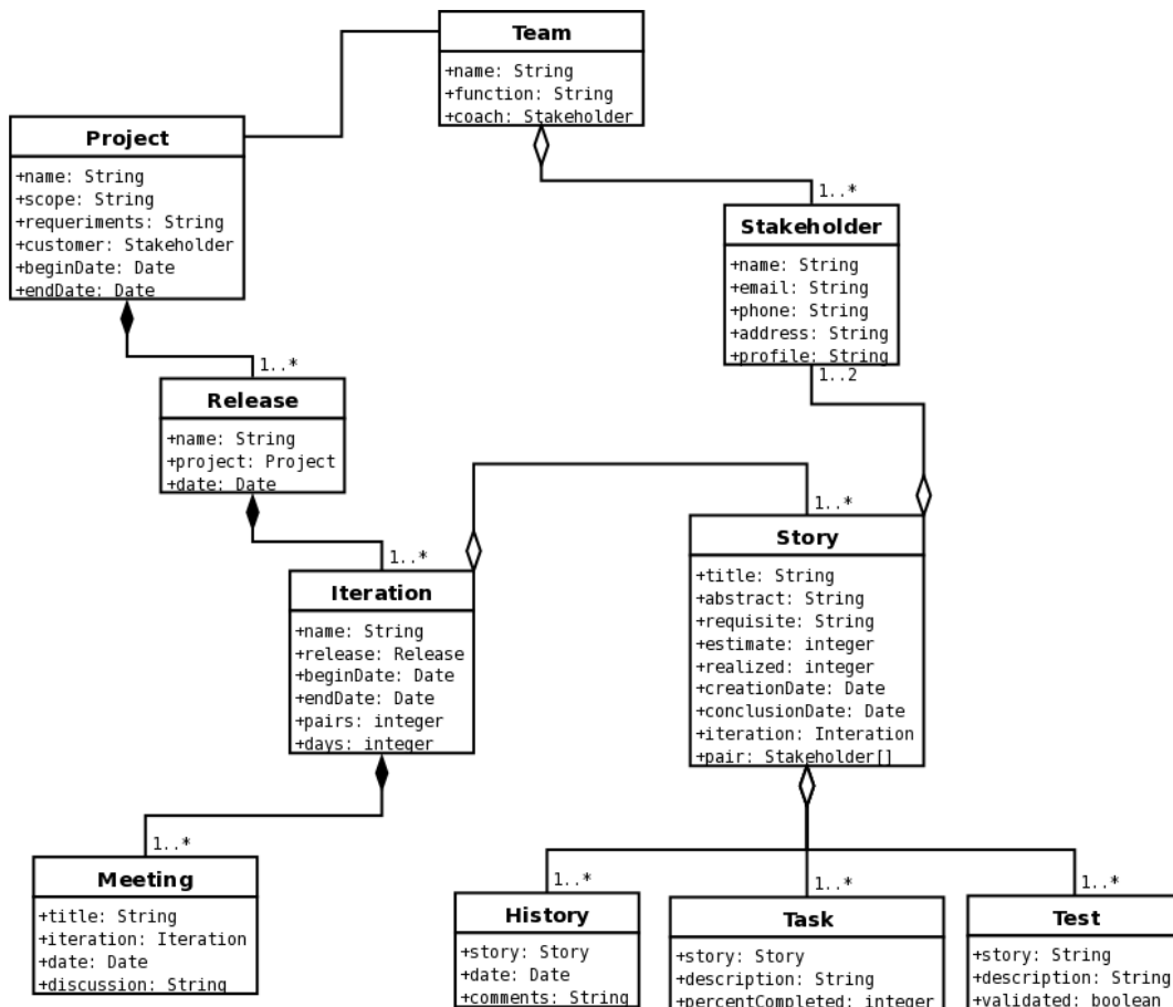
Figura 14: Metamodelo da metodologia XP (Desenvolvido pelo autor)
