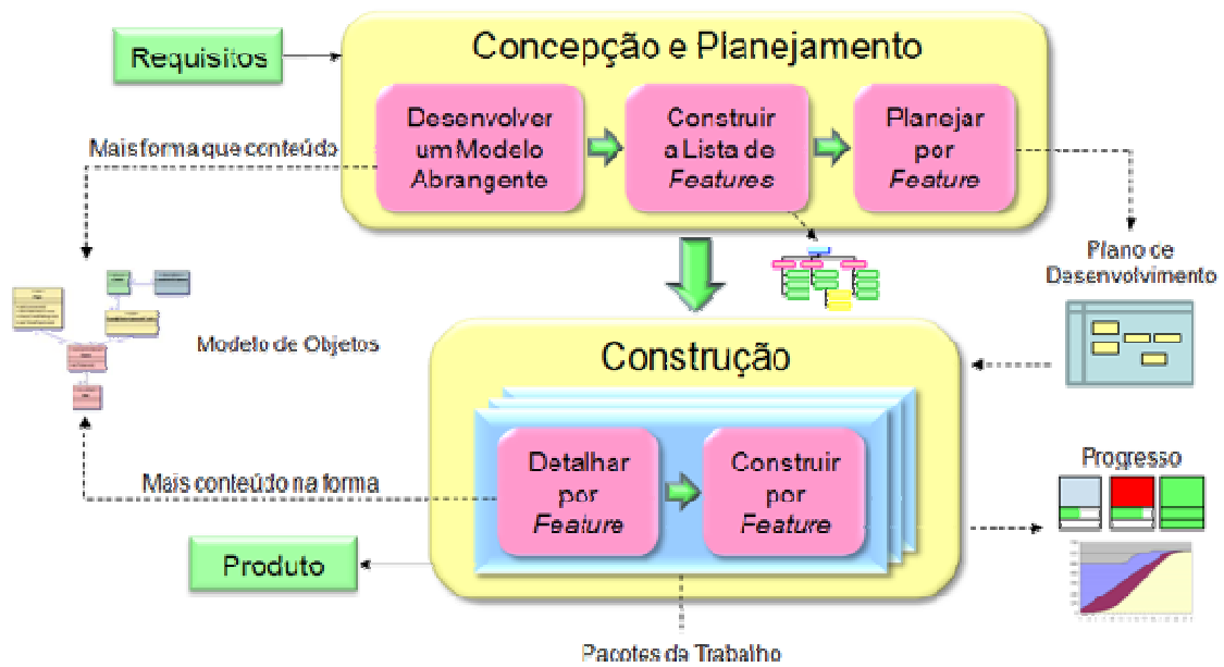
Figura 3: Processo da metodologia FDD (FDD, 2010)
