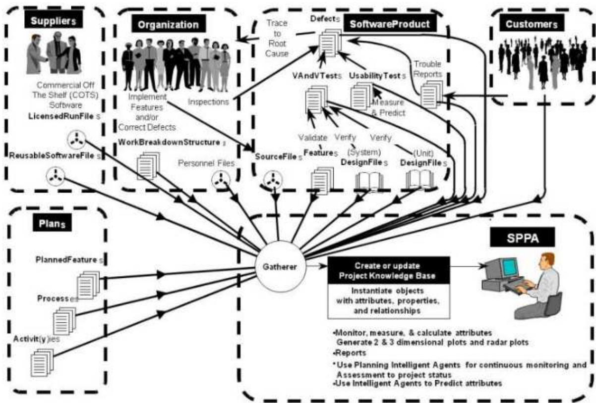
Figura 9: Estrutura do SPPA (CHANG et al., 2009)
