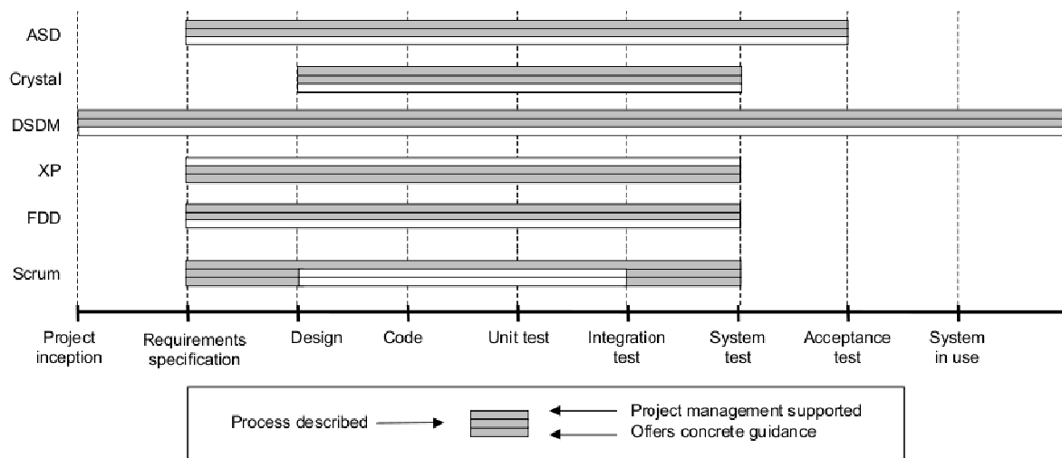
Figura 5: Perspectivas para metodologias ágeis (ABRAHAMSSON et al., 2003)
