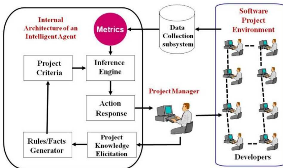
Figura 11: Arquitetura dos agentes inteligentes (CHANG et al., 2009)
